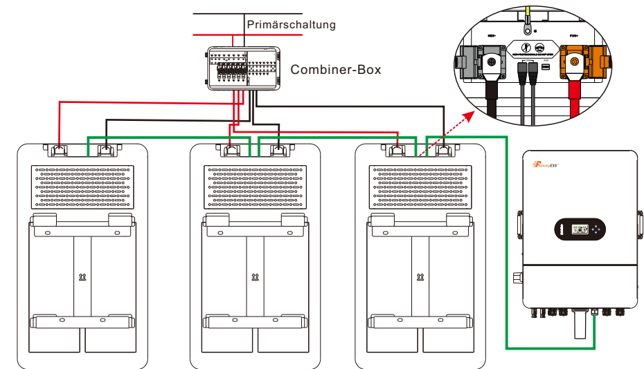
Abbildung 1: Die Parallelschaltung von drei Akkupacks
